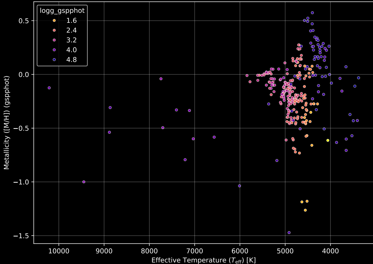
APOGEE DR17 Field: [135-24_btx] Stellar Population Parameters (n= 298)
